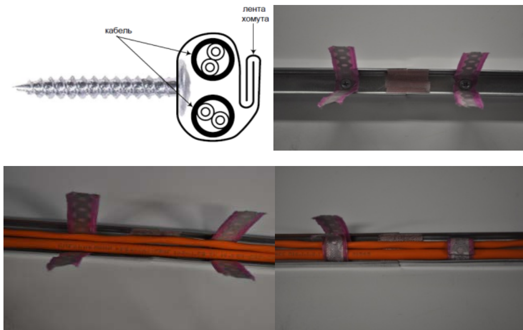
Рис. 4. Порядок установки дюбель-хомута КФСТ.735322.041
